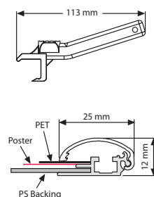
Levertool / Öffnungsapparat ARTICLE: UYUP047000
